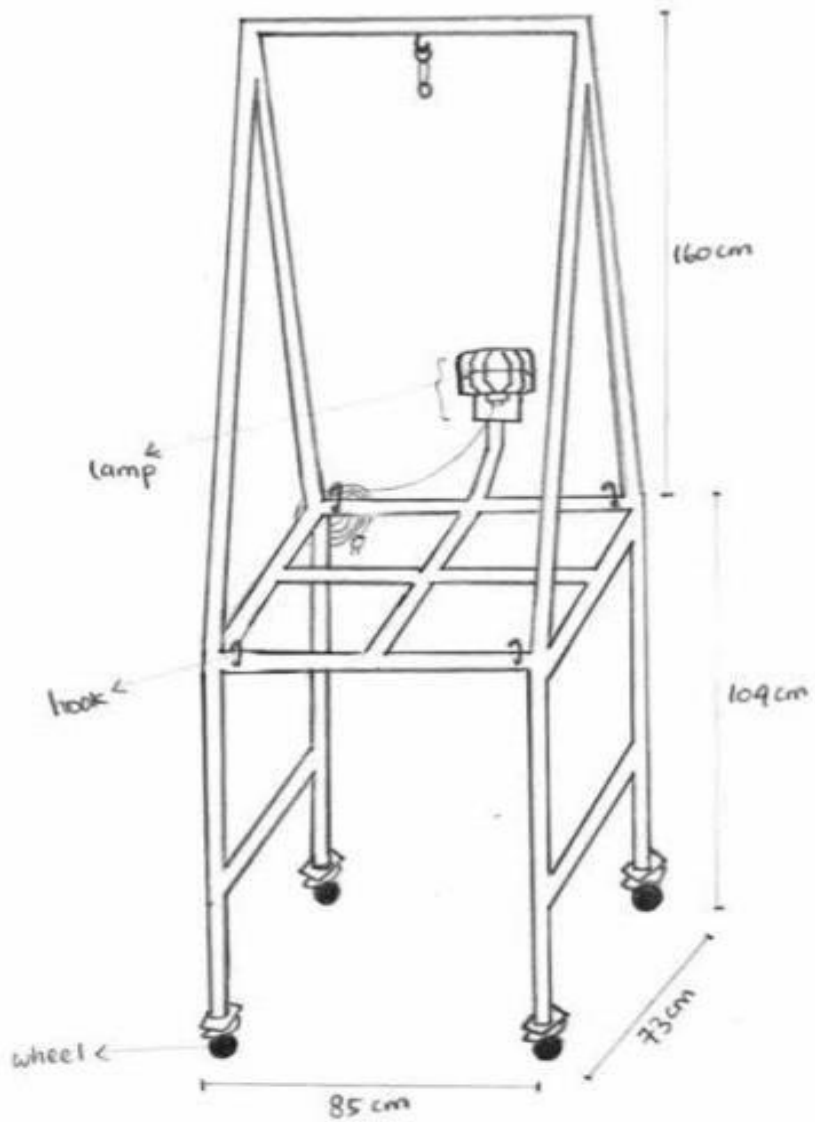
Gambar 2.3 Bingkai Yang Dapat Berpindah
